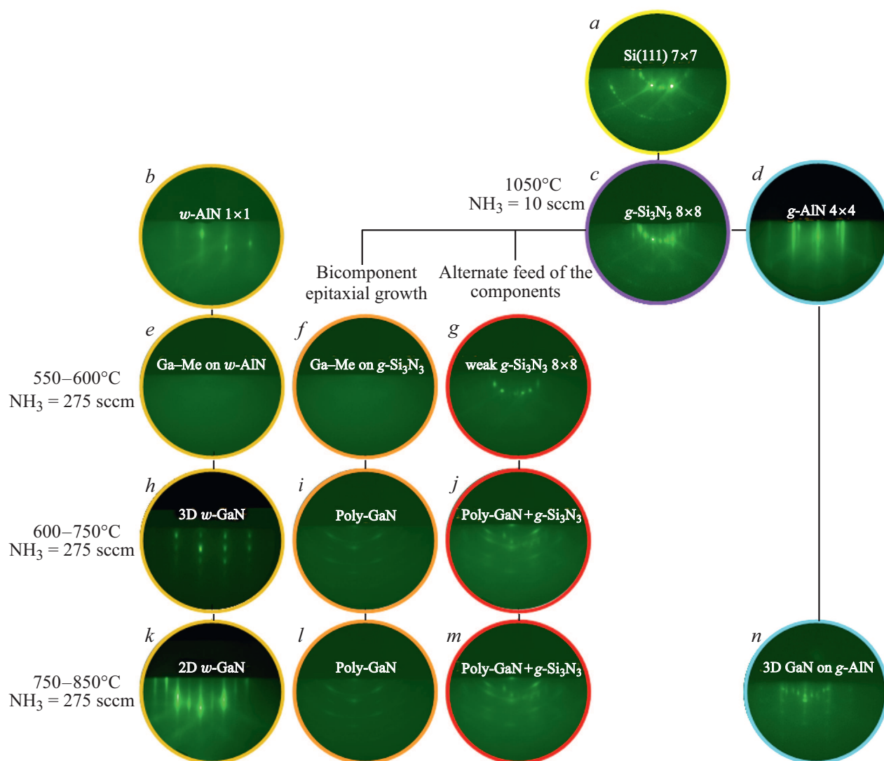
Рис. 1. Сравнительная схема эволюции дифракционных картин в процессе синтеза GaN на поверхностях q -Si 3 N 3 , q -AlN и w -AlN.
