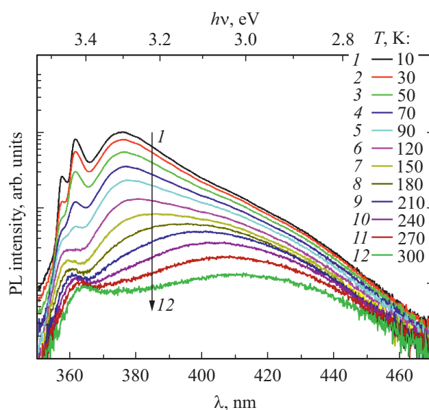
Рис. 3. Спектры ФЛ GaN на g\text{-AlN}/g\text{-Si}_3\text{N}_3/\text{Si}(111) при различных температурах.
